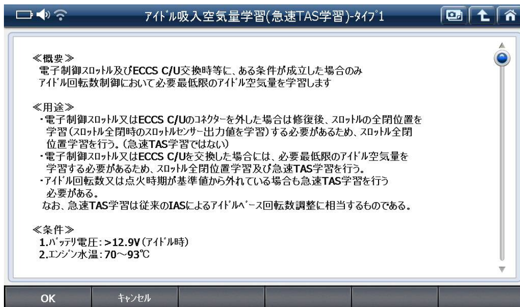
〈図:アイドル吸入空気量学習(急速 TAS 学習)-タイプ1の実行〉
