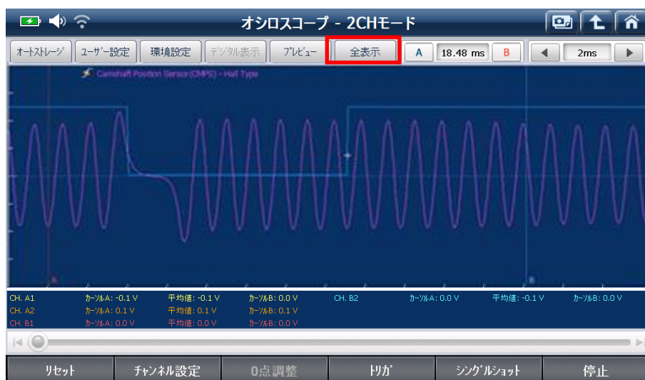
[全表示 - CMP+CKP 同期]
