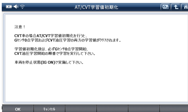
[作業サポート - 説明画面]
