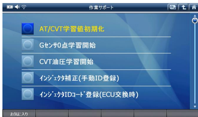
[作業サポート - 項目表示]
