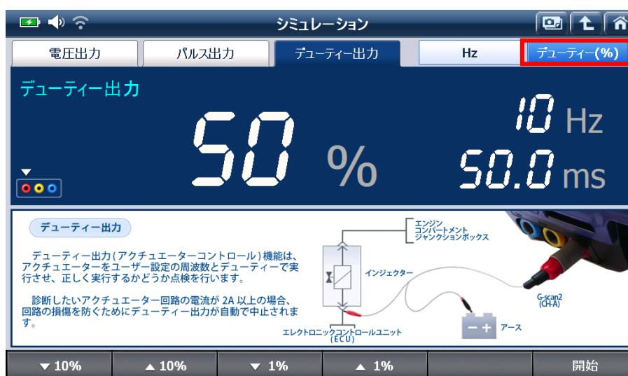
[シミュレーション デューティー出力(%)画面]
