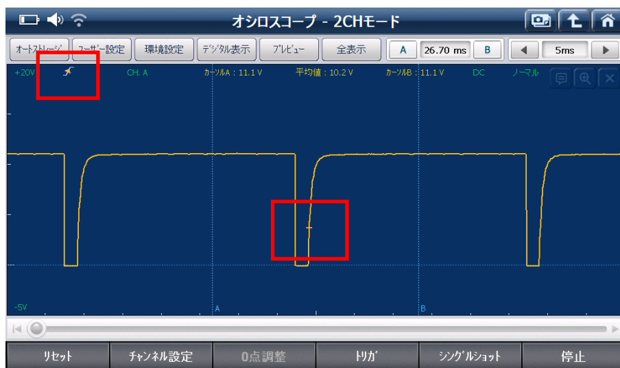
[トリガ設定 立ち上がり画面]
