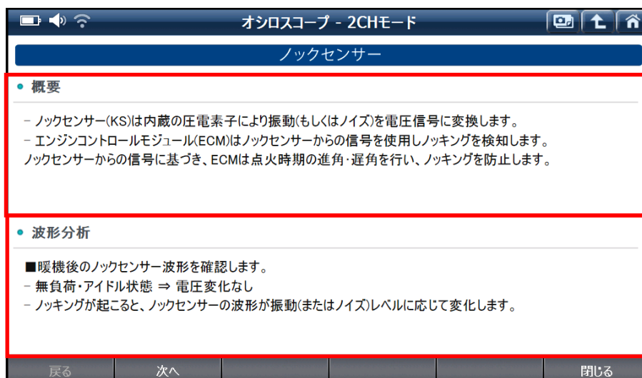
[オシロスコープ [ヘルプ]アイコン選択画面]
