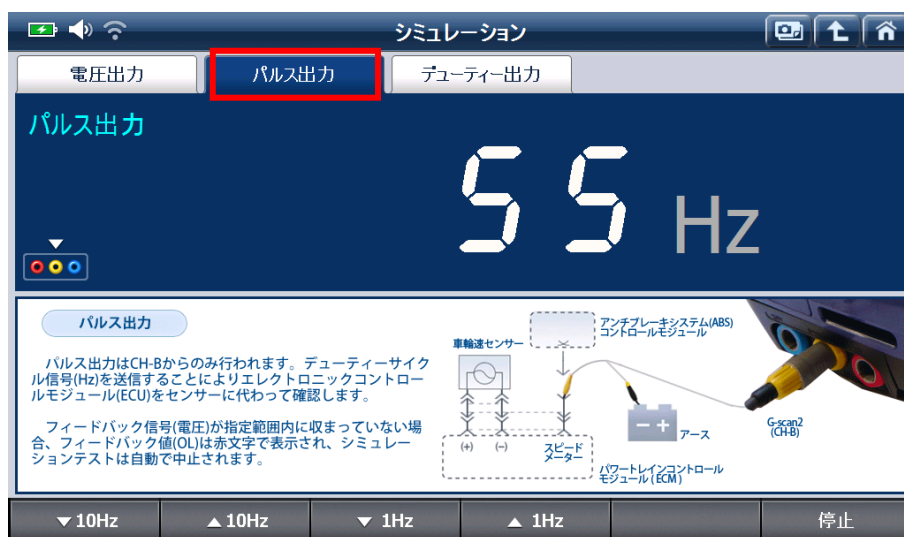
[シミュレーション パルス出力画面]
