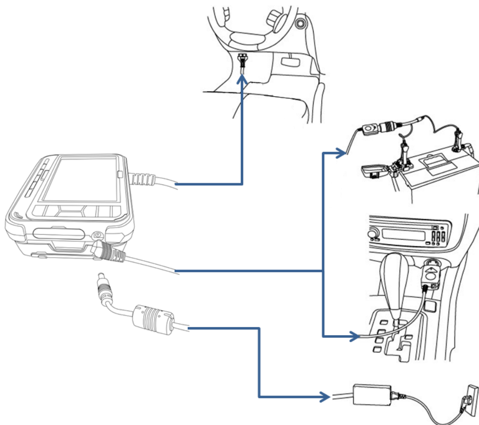
[G-scan2への電源供給]
