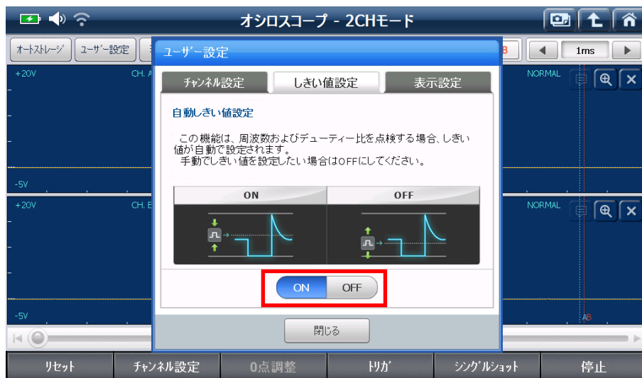
[オシロスコープ しきい値設定画面]
