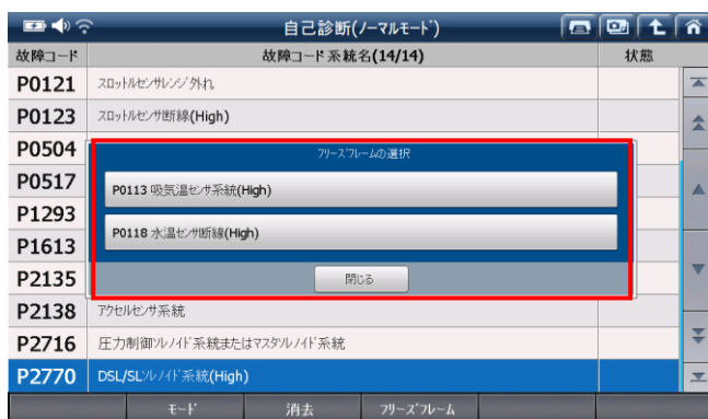
[フリーズフレーム 選択画面]
