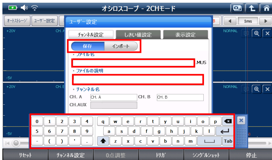
[オシロスコープ 設定保存画面]
