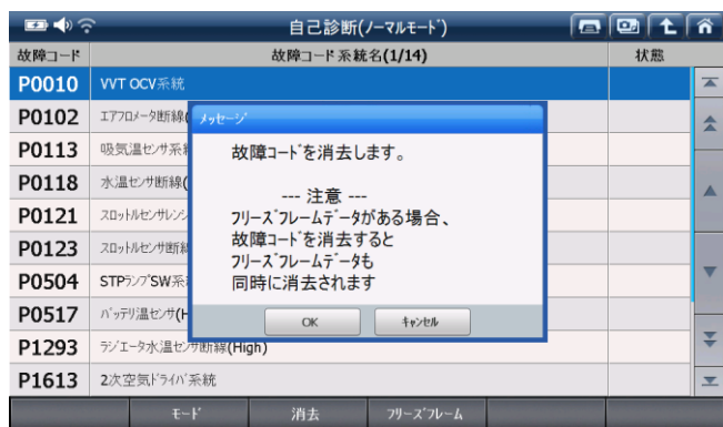
[自己診断 - 消去確認メッセージ]
